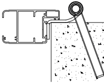
AMI7 - BATTUTA CONTRO MARMO
