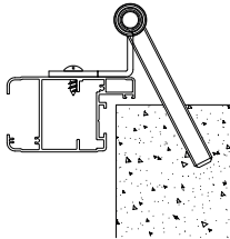
AMI8 - ZOCCOLO A SFIORO
