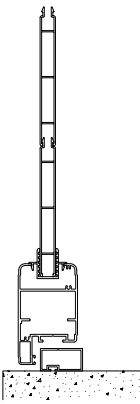
AMI7 - BATTUTA CONTRO MARMO
