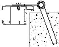
AMI - BANDELLA A CROCE CON CARDINE DA 90 mm
