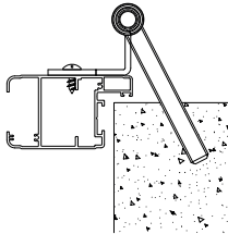
FM3 - BANDELLA A GOMITO FESSA CON CARDINE DA 90 mm
