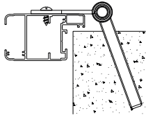
FM1 - BANDELLA A CROCE CON CARDINE DA 90 mm
