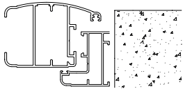
M13 - TELAIO A "L" NORMALE
