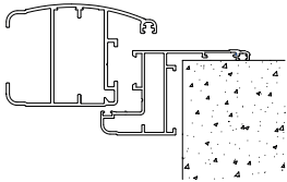
M11 - TELAIO "Z" NORMALE FALDA DA 40 mm
