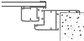
ST3 - TELAZIO "Z" MAX FALDA 50 mm
