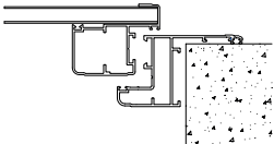
ST1 - TELAIO "Z" NORMALE FALDA DA 40 mm
