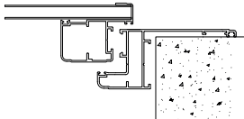
ST2 - TELAIO "Z" NORMALE FALDA DA 65 mm
