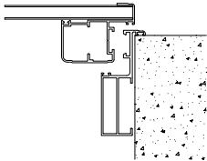
ST19 - ANTA A SFIORO
