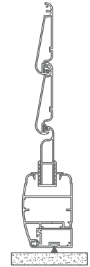
AR10 - NODO INFERIORE ANTA A SFIORO
