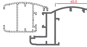
AR2 - TELAIO "L" NORMALE
