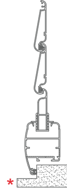
AR8 - NODO INFERIORE BATTUTA MARMO
